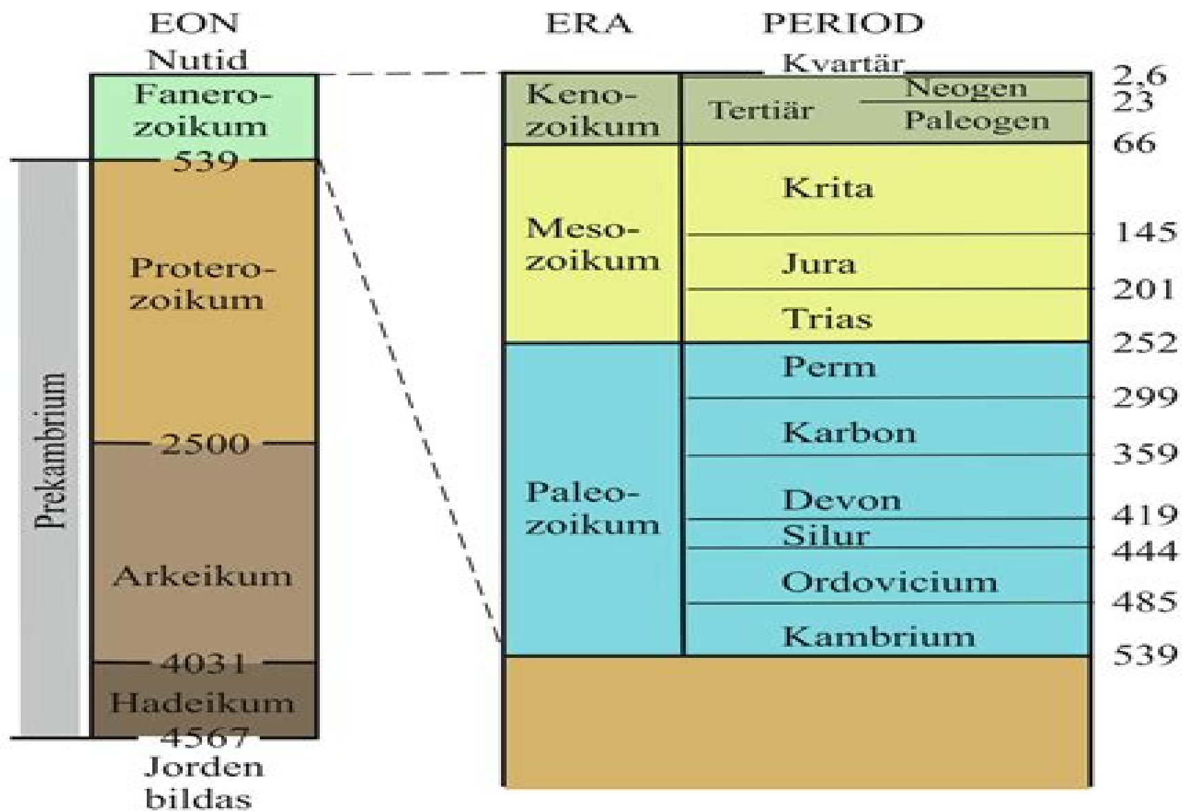
Geologisk tidsskala med åldrar i miljoner år efter International Stratigraphic Chart (International Commission on Stratigraphy, IUGS, 2023)
