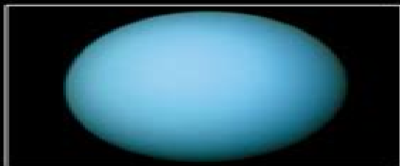
Uranus
