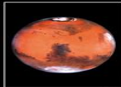
Mars
