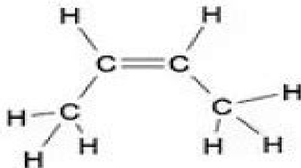
cis-2-butene
